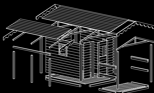
Esploso casetta con tettoia e veranda
